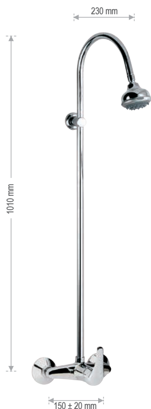
F 36 2 Gruppo doccia con colonna lusso e soffione doccia art. 358GR, 4 getti, anticalcare.
