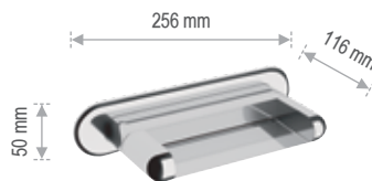
359 NC Soffione doccia con bordi arrotondati. C.p. brass shower head with rounded corners.
