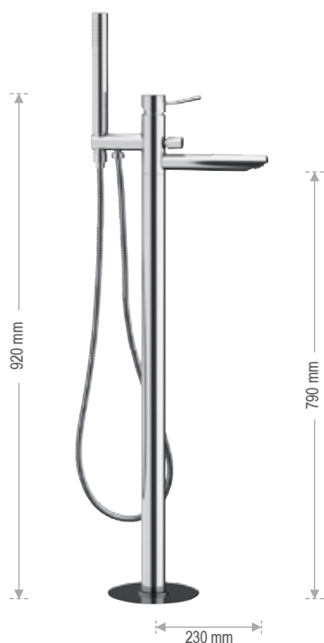
N 08 Miscelatore vasca da pavimento con deviatore e kit doccia.
