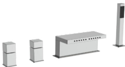
S 06 3 Miscelatore monocomando bordo vasca con deviatore, bocca con effetto multigetto e doccetta in ottone cromato. Single lever deck bath/shower mixer with diverter, spout with multijets effect and c.p. brass hand shower.
